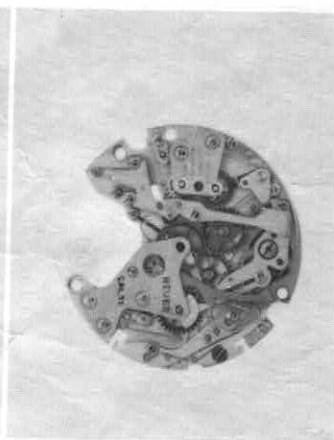
MECANISME DE CHRONOGRAPHE
